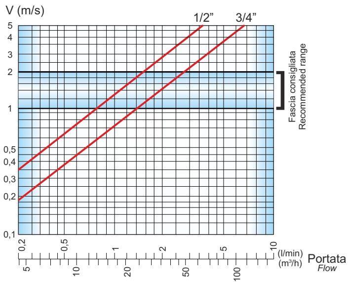
Diagramma velocità di circolazione Flow velocity diagram
