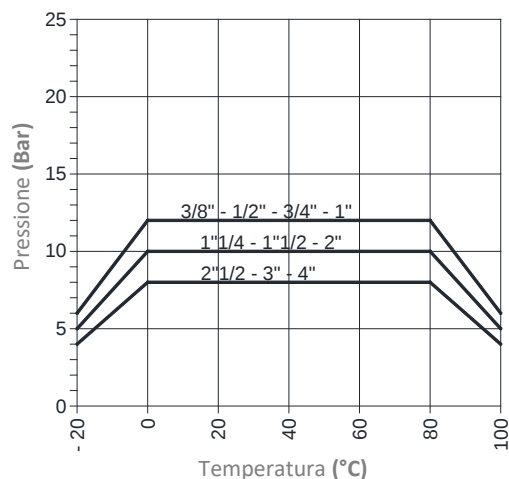
Diagramma 2: Pressione/temperatura.
